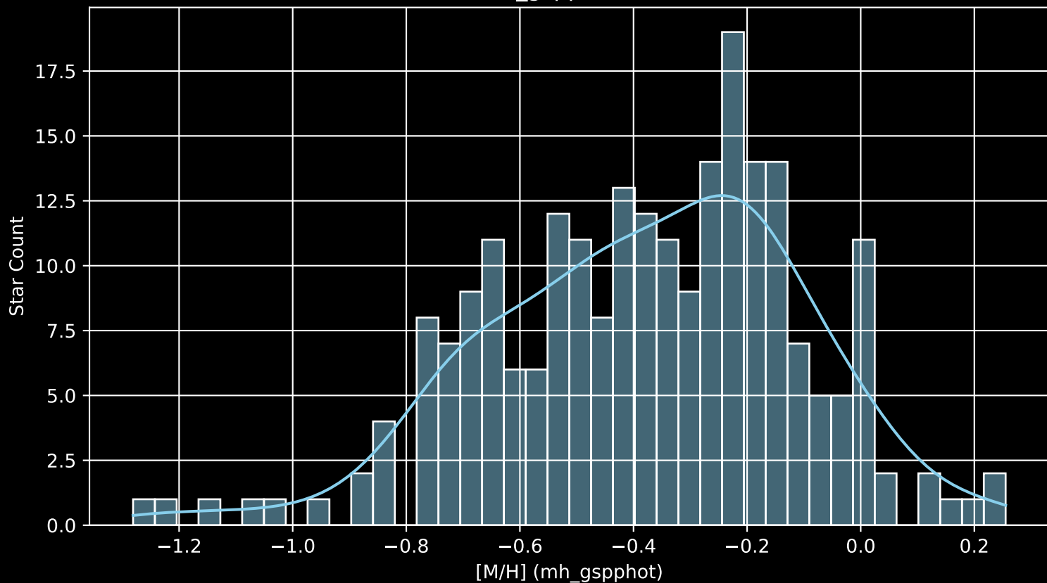
GALAH DR4 Field: [8613] [M/H] (mh_gspphot) (n= 232)
