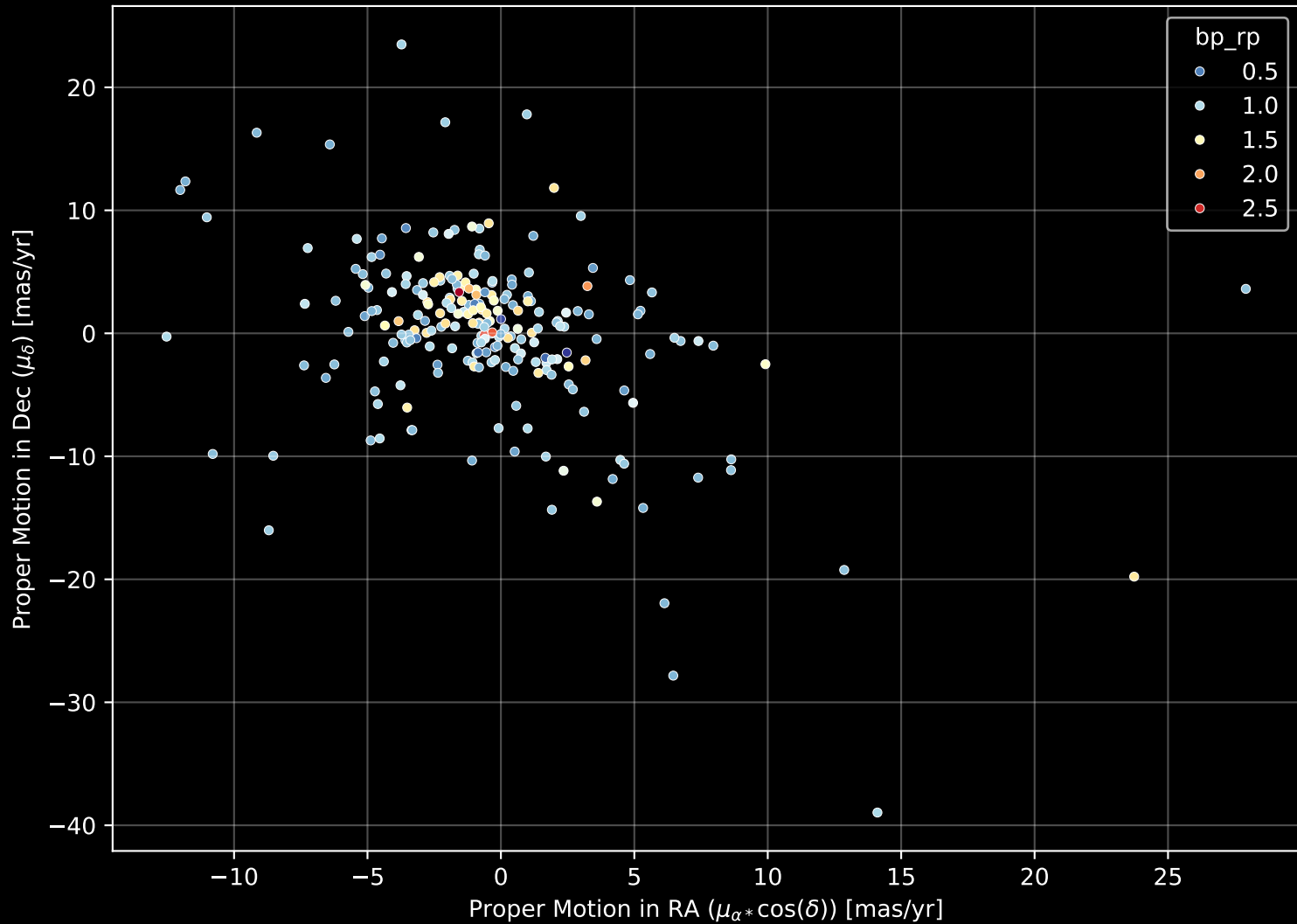
GALAH DR4 Field: [8613] Proper Motion Diagram (n= 232)
