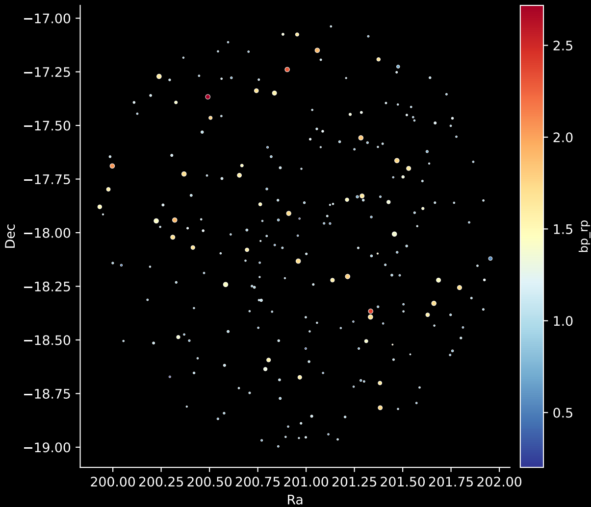
GALAH DR4 Field: [8613] Stars: 232
