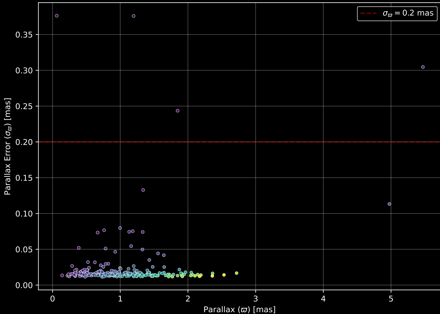
GALAH DR4 Field: [8613] Parallax Quality (n= 232)
