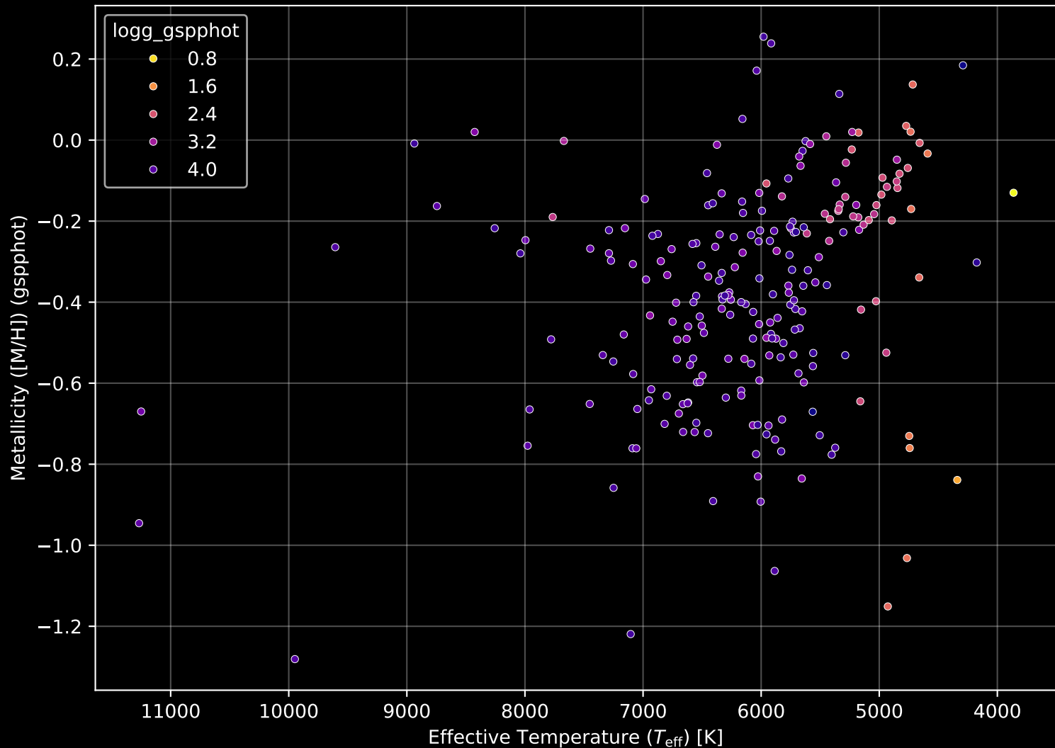
GALAH DR4 Field: [8613] Stellar Population Parameters (n= 232)
